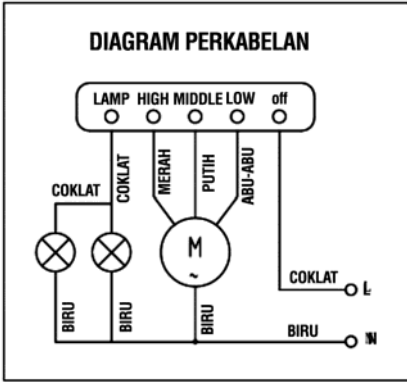
Motor tunggal
