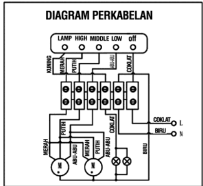
Motor ganda
