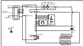
DIAGRAM PERKABELAN – MODEL DPDT, DENGAN ELCB, TANPA POMPA (HANYA UNTUK MODEL VIETNAM)
