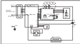
DIAGRAM PERKABELAN – MODEL DPDT DENGAN ELCB, POMPA DC
